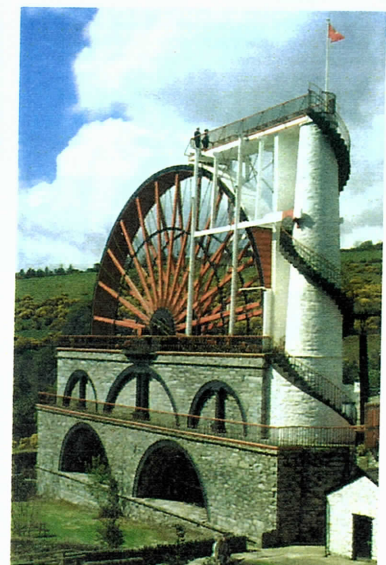
La "Lady Isabella" à Laxey. La plus grande roue à eau du monde qui soit encore en état de marche
